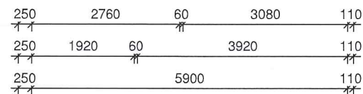
eerste verdieping
